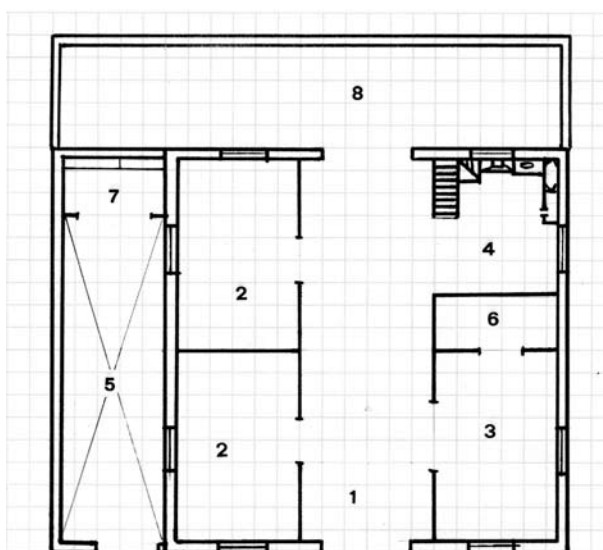
Planta baixa
