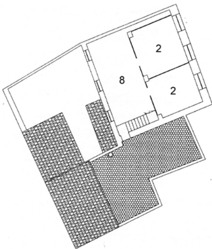
Plànol de la distribució actual de l'hort Mandarí: 1.- Pas-sadís, 2.- Habitacions, 3-4.- Cuina menjador, 5.- Sala, 6.- Corral, 7.- Quadra, 8.- Cambra.
